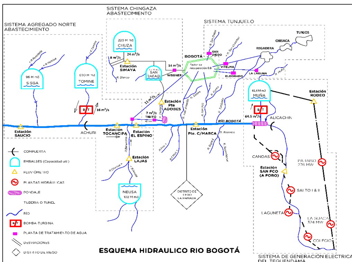
Figura 17. Esquema Hidráulico Río Bogotá Fuente. EAB –CAR. Adaptado por IDIGER. 2015
