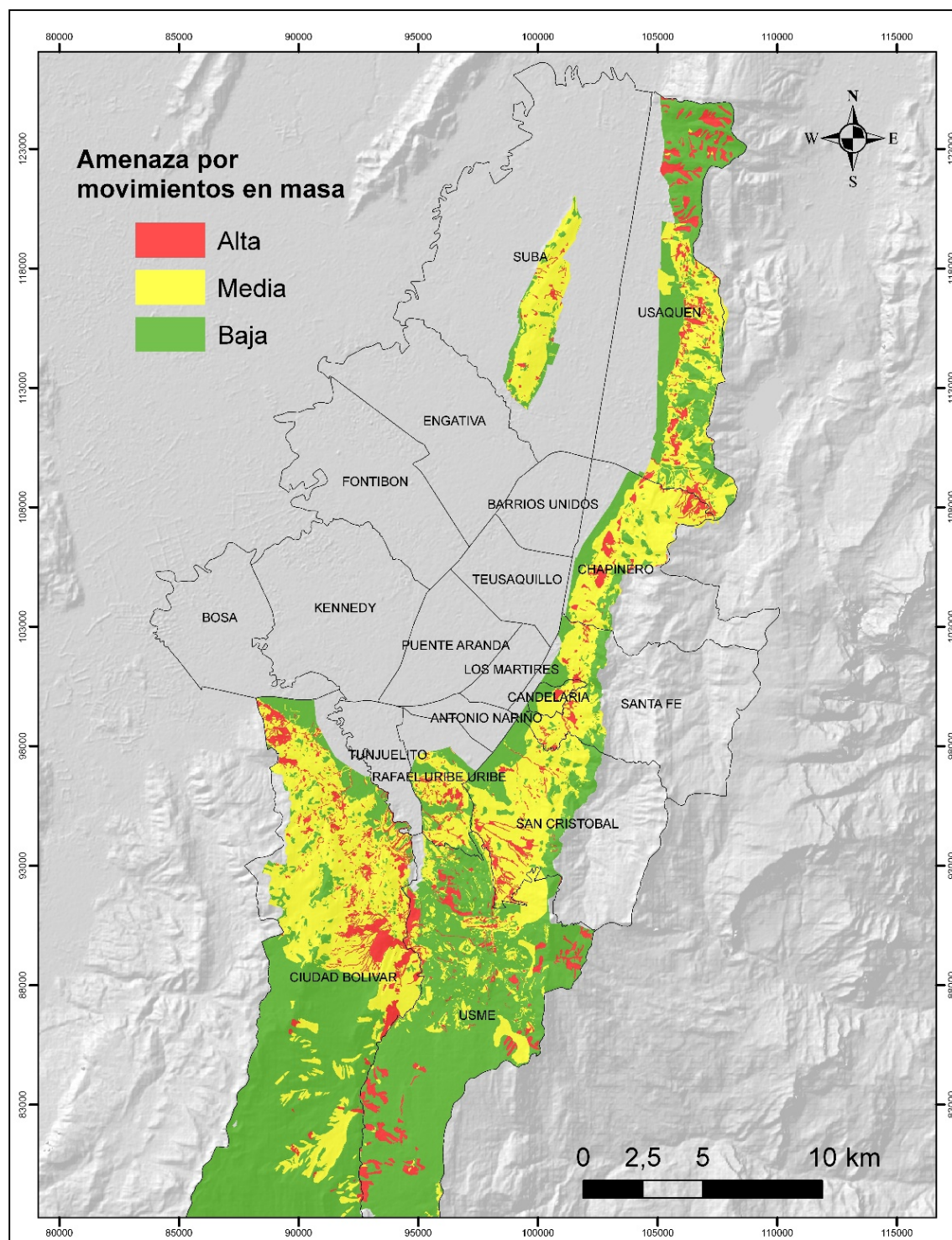
Figura 12. Plano de amenaza por movimientos en masa. En rojo se ilustran las zonas de amenaza alta. Plano Normativo Decreto 190/2014 Fuente. IDIGER. 2017
